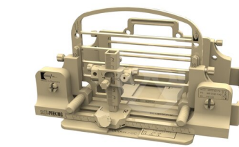
Urządzenie do biopsji piersi wykonane z materiału SUSTAPEEK MG
